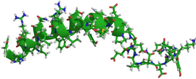
Şekil.1. Nöropeptid Y'nin Yapısı [109]
